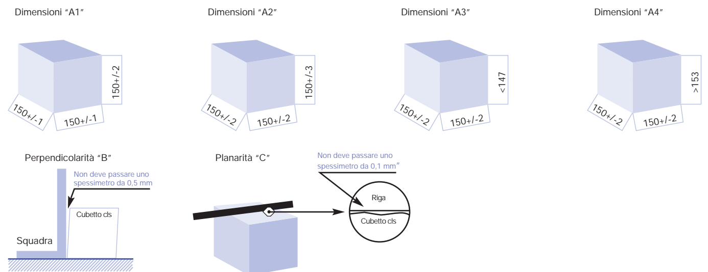
Verifiche dimensionali sui cubetti di calcestruzzo
