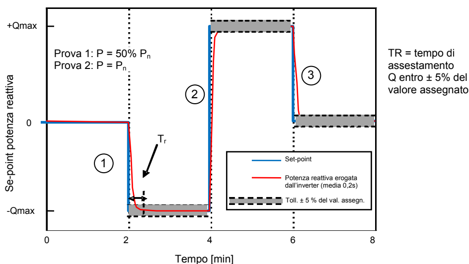
Figura 26 – Misura del tempo di risposta a variazioni a gradino del set-point assegnato per la potenza reattiva
